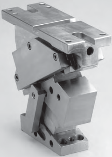
NAC075-20 NAAMS Aerial Cam
